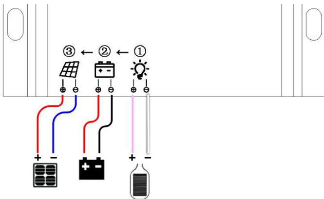
24160 24200 Wiring Diagram:
