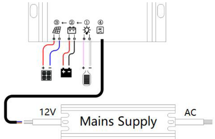
24160-AC Wiring Diagram:
